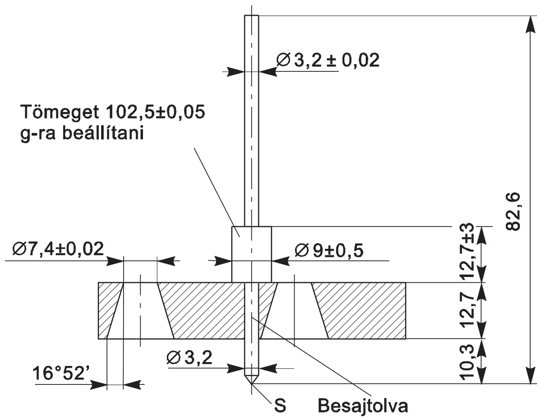
4. ábra: Penetrométer
