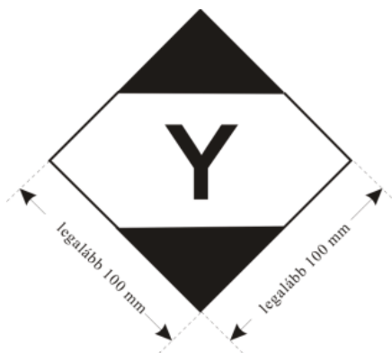
Az ICAO Műszaki Utasítások 3. Rész, 4. fejezetének megfelelő, korlátozott mennyiséget tartalmazó küldeménydarabok jelölése
