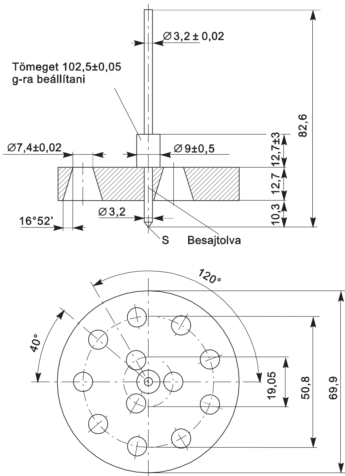
4. ábra: Penetrométer
